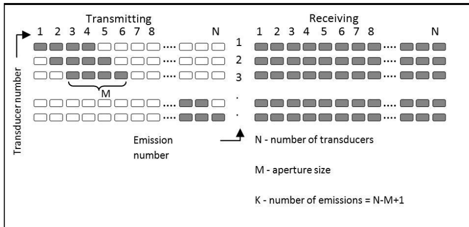
Fig.5 Scheme of STA mode.
